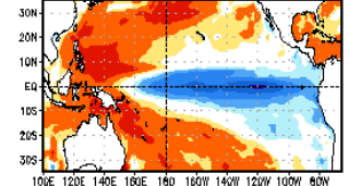
Nov–Dec 2024/2025
