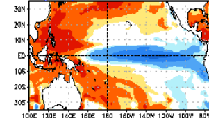
Aug–Sep–Oct 2024
