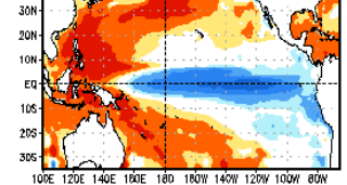
Oct–Nov–Dec 2024
