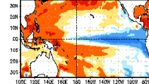
Jul–Aug–Sep 2024
